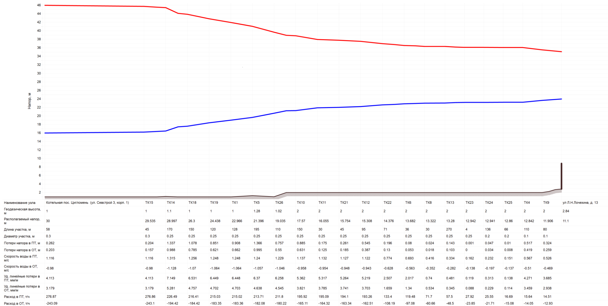
Рисунок 30 - Существующий гидравлический режим тепловых сетей от котельной пос. Цигломень, ул. Севстрой 3, корп. 1
