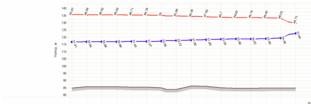
Рисунок 25 - Пример пьезометрического графика
