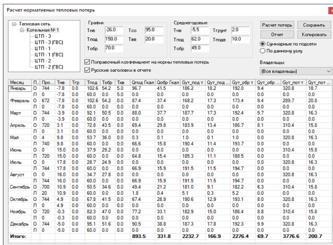
Рисунок 24 - Результаты расчета потерь тепловой энергии через изоляцию и с утечками теплоносителя
